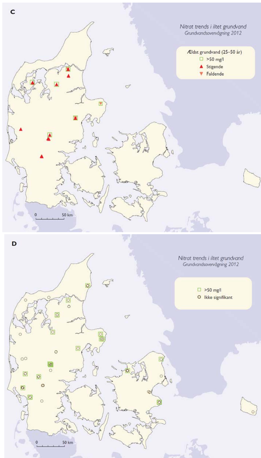
Figur 15. Geografisk fordeling og gruppering af statistiske nitrattrend analyser i 152 indtag i iltet dateret grundvand: A: Signifikante nitrattrends i yngst grundvand, B Signifikante nitrattrends i medium grundvand, C: Signifikante nitrattrends i ældst grundvand og D: ikke signifikante nitrattrends (modificeret efter Hansen m.fl., 2012). Figurens første to dele se forrige side.
