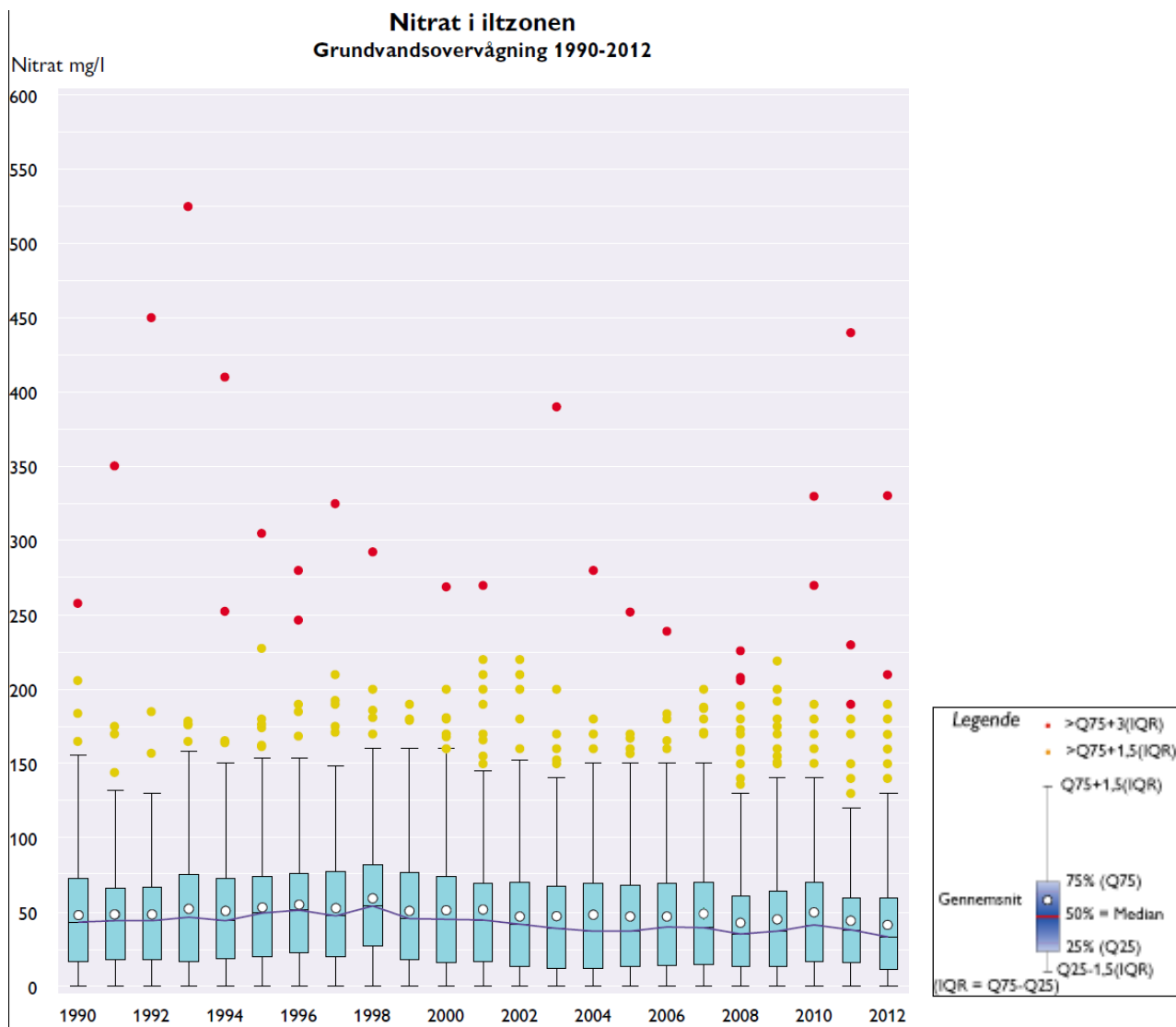
Figur 10. Udviklingen i iltet (ilt >1 mg/l) grundvands nitratindehold, GRUMO 1990 - 2012.
