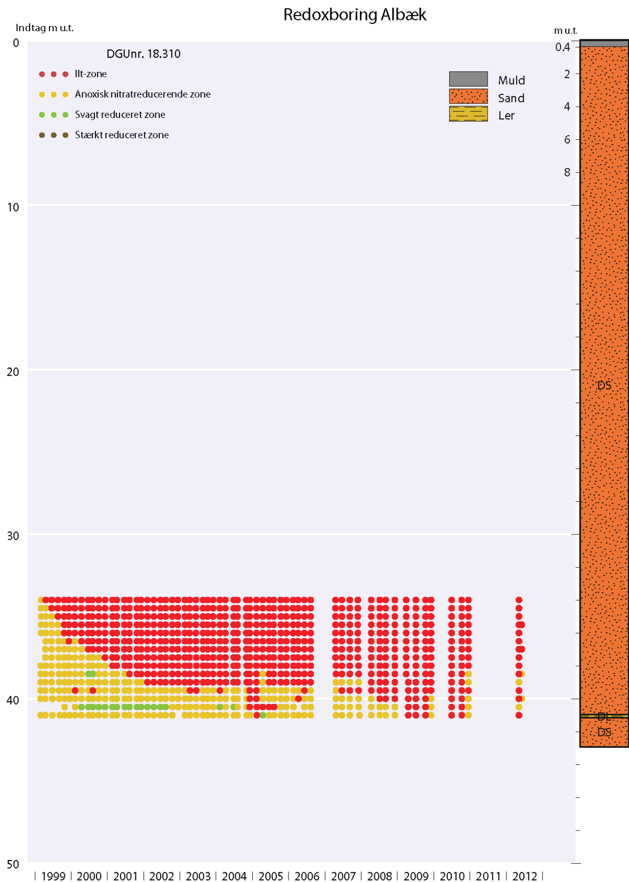
Figur 16. Redoxzoner 33-43 m u.t. for redoxboring DGU nr. 18.310, Albæk, v. Sæby 1999-2012. Grundvandsspejl i ca. 15,5 m u.t. Den geologiske lagserie er vist på figuren længst til højre.
