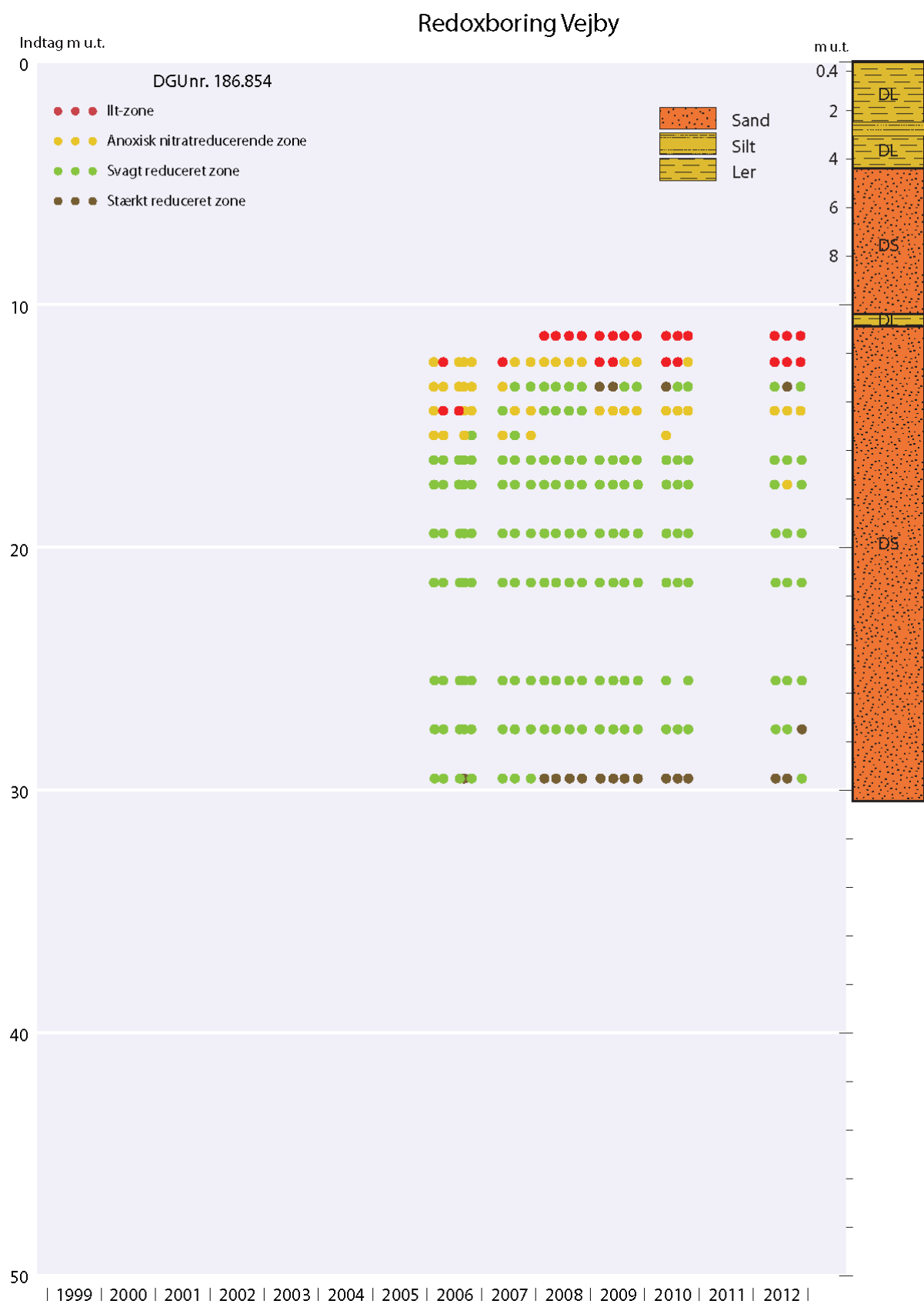
Figur 20. Redoxzoner 13 - 30 mu.t. for redoxboring DGU nr. 186.854 og 186.855, Vejby, Nordsjælland, 2006-2012. Grundvandsspejl i ca. 10 m u.t. Den geologiske lagserie er vist til højre.
