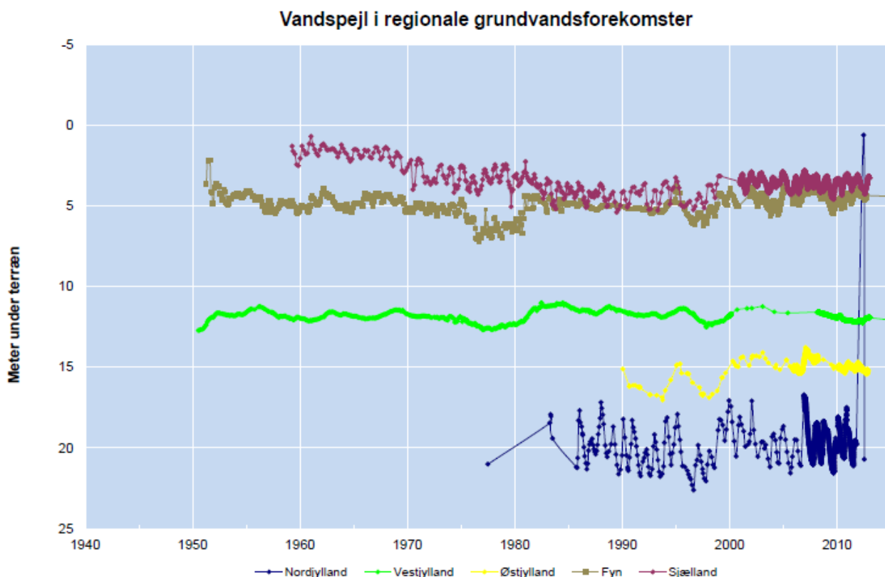
Figur 61. Pejletidsserier (vandstand i m u.t.) for regionale grundvandsforekomster.
