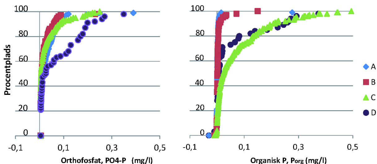
Figur 23. Indholdet af Orthofosfat-P ( \text{PO}_4\text{-P} ) og Organisk bundet fosfor ( \text{P}_{\text{org}} ) opdelt efter vandtype, jf. tabel 3 og side 40. Vandtype A og B indeholder nitrat, mens vandtype C og D er reducerede.
