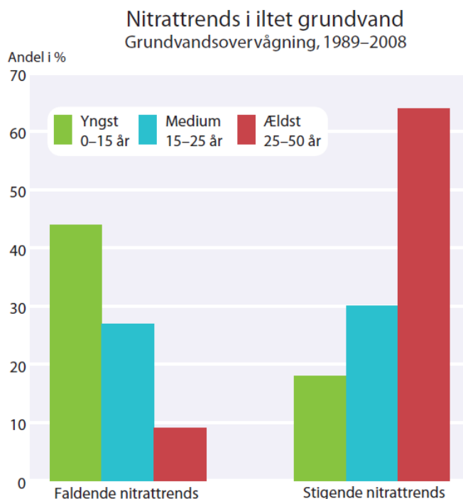
Figur 14. Andel af statistisk signifikante (95 % konfidens) stigende og faldende nitrattrends i grundvandet, inddelt i 3 aldersgrupper (modificeret efter Hansen m.fl., 2011).
